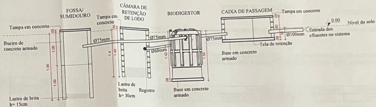
CORTE ESQUEMÁTICO 1/50
