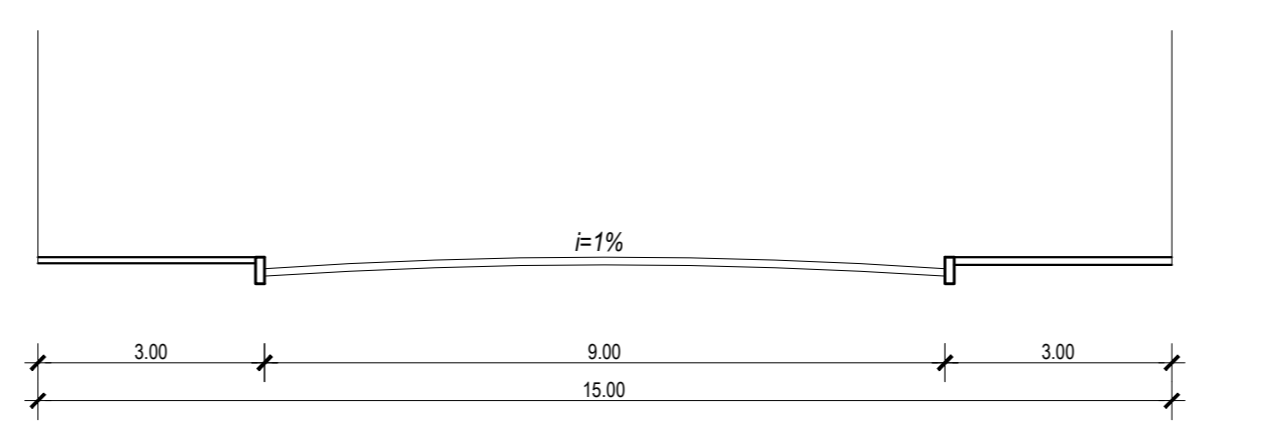
Corte Transversal - Ruas Escala: 1/100
