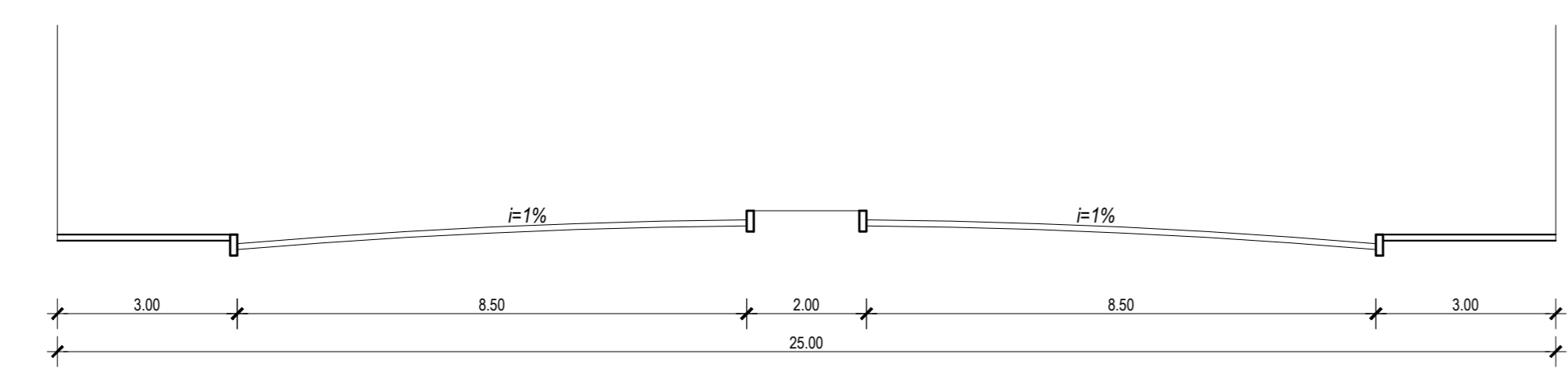
Corte Transversal - Avenida Principal Escala: 1/100
